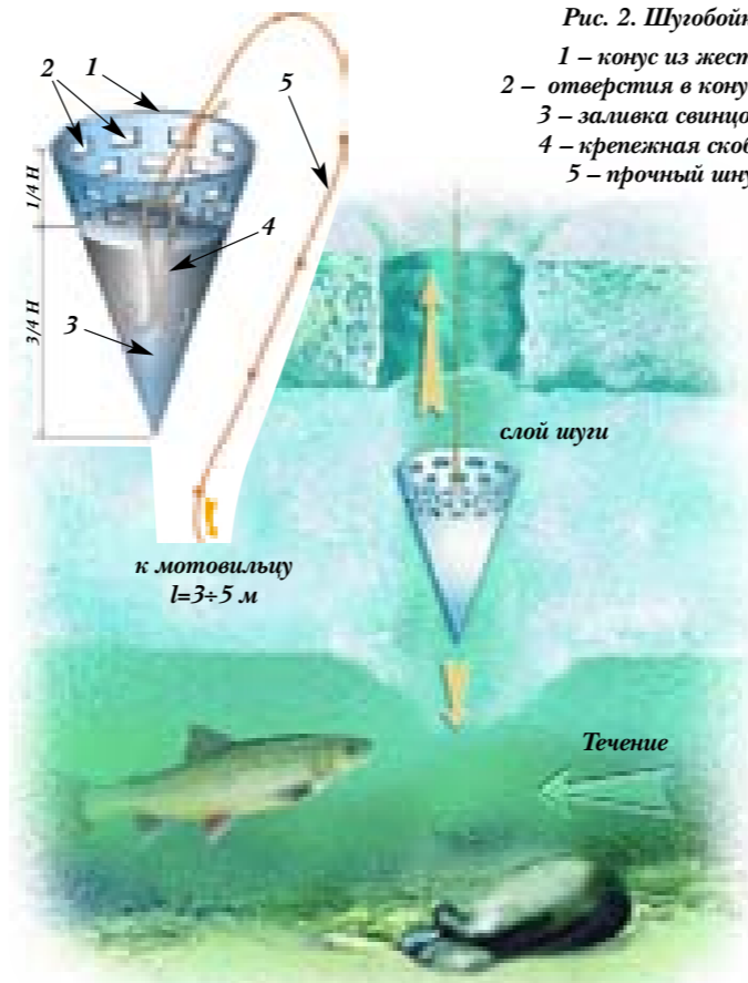
Рис. 2. Шугобойка:
